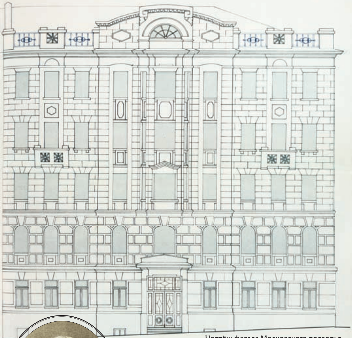
Чертёж фасада Московского подворья Саровской Успенской пустыни. ЦГАРМ
